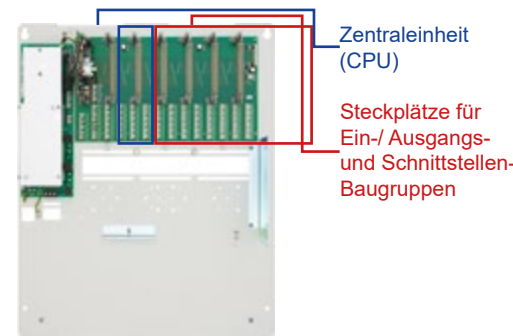
Securitel 500-M im Gehäuse H 550 6 Steckplätze
